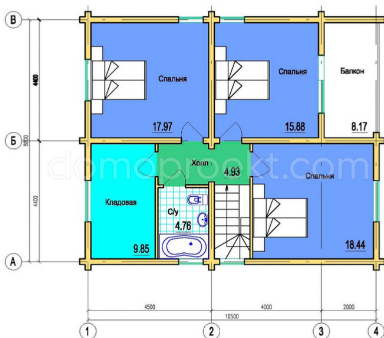
План 2 этажа
